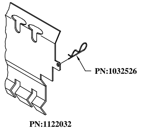
Spacer
